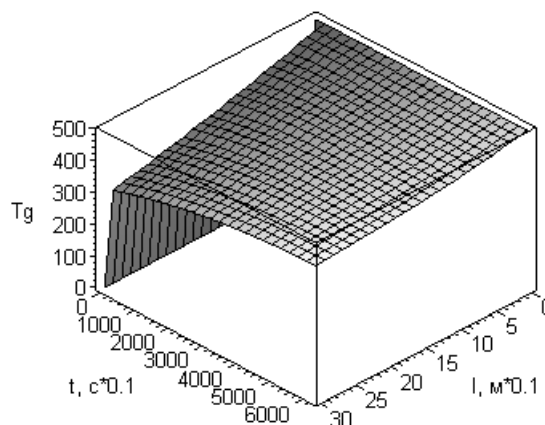
Рис. 3. Зависимость температуры сушащего газа T_g от времени и длины барабана
