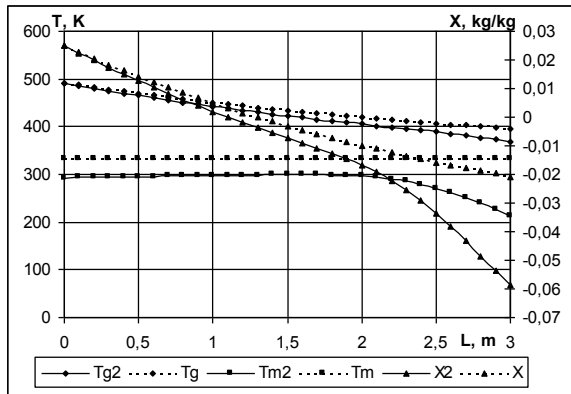
Рис. 12. Графики решения систем M\_L\_YP\_RV2 ( X , T_g , T_m ) и системы M\_LT\_RV2 ( X_2 , T_{g2} , T_{m2} )
