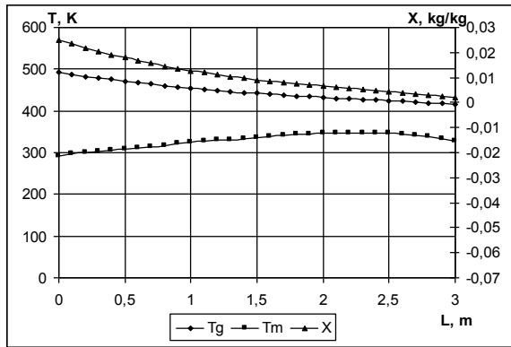
Рис. 6. Графики решения системы M_LT_RV1
