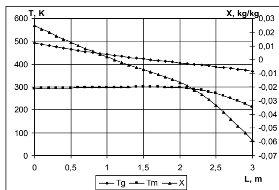
Рис. 5. Графики решения системы M_{LT\_RV2}
