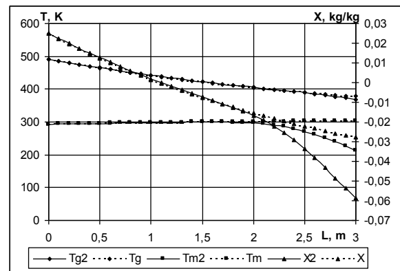
Рис. 11. Графики решения систем M_{L\_YP\_RV2} ( X , T_g , T_m ) и системы M_{LT\_RV2} ( X_2 , T_{g2} , T_{m2} )
