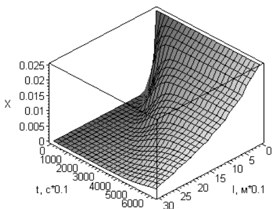
Рис. 2. Зависимость влажности материала X от времени и длины барабана
