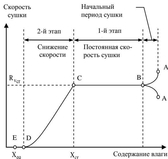
Рис. 1. Типичная кривая скорости сушки
