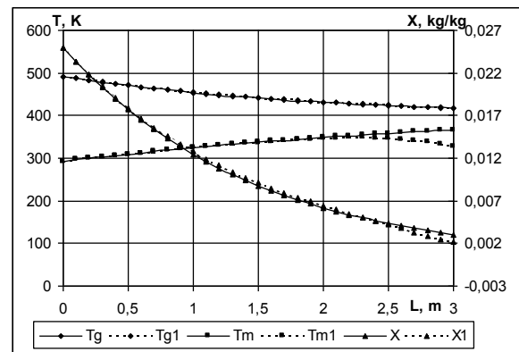
Рис. 10. Графики решения систем M_{L\_YP\_RV1} ( X , T_g , T_m ) и системы M_{LT\_RV1} ( X_1 , T_{g1} , T_{m1} )
