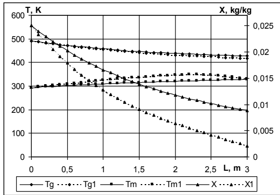
Рис. 9. Графики решения систем M_{TY\_RV1} ( X , T_g , T_m ) и системы M_{LT\_RV1} ( X_1 , T_{g1} , T_{m1} )
