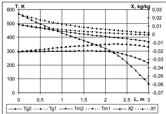
Рис. 7. Графики решения систем M_LT_RV1 ( X_1, T_{g1}, T_{m1} ) и системы M_LT_RV2 ( X_2, T_{g2}, T_{m2} )
