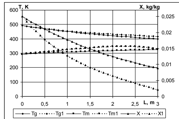
Рис. 8. Графики решения систем M_LT_RV1 ( X_1, T_{g1}, T_{m1} ) и системы M_TP_RV1 ( X, T_g, T_m )
