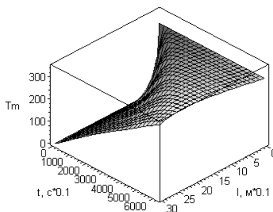
Рис. 4. Зависимость температуры материала T_m от времени и длины барабана
